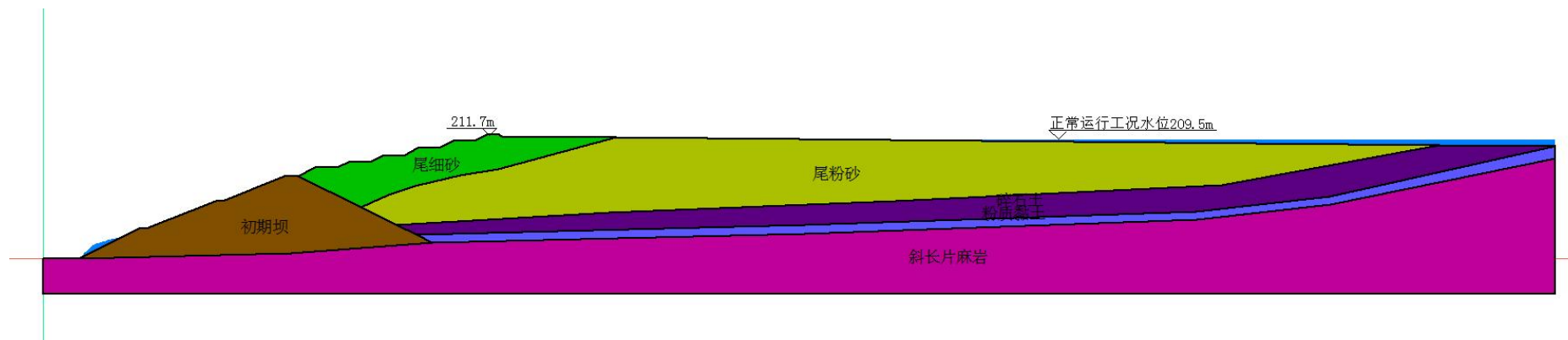
图 3.2-3 尾矿库现状正常运行工况 209.5m 水位加荷载
