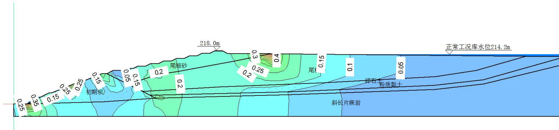
图 3.2-14 尾矿库末期正常运行工况坝体内部水力梯度计算结果云图
