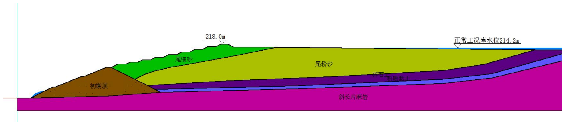
图 3.2-13 尾矿库末期正常运行工况 214.2m 水位加荷载
