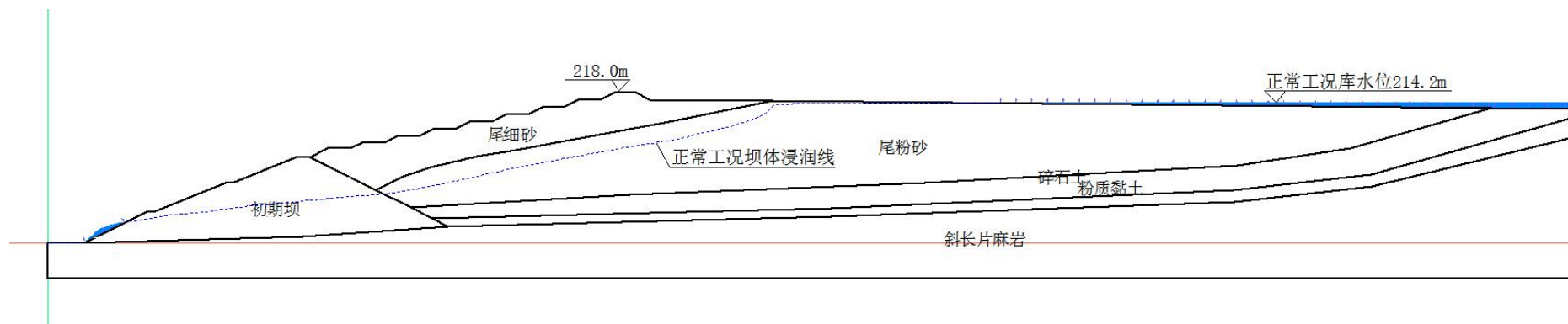
图 3.2-15 尾矿库末期正常运行工况坝体内部浸润线计算结果云图
