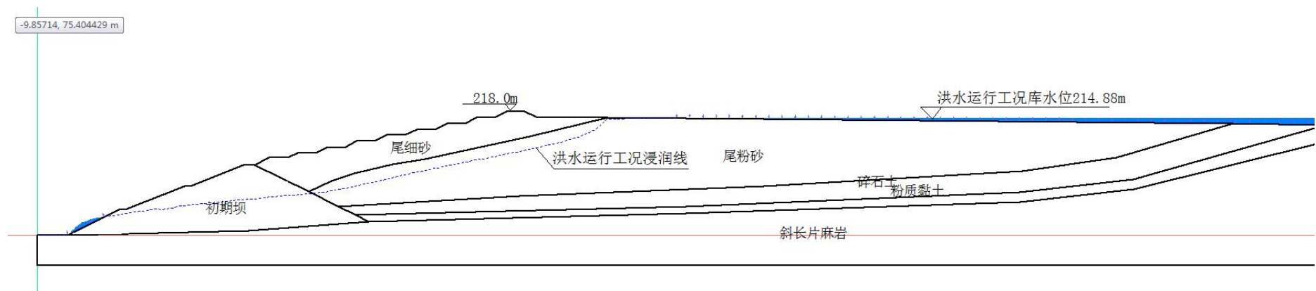
图 3.2-18 尾矿库末期洪水运行工况坝体内部浸润线计算结果云图
