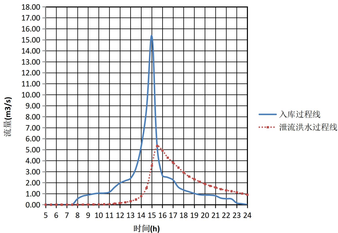
图 3.3-8 尾矿库调洪验算过程曲线图
