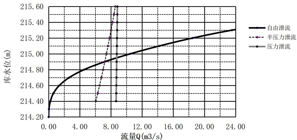
图 3.3-10 排水斜槽排水系统库水位与泄流量关系曲线图
