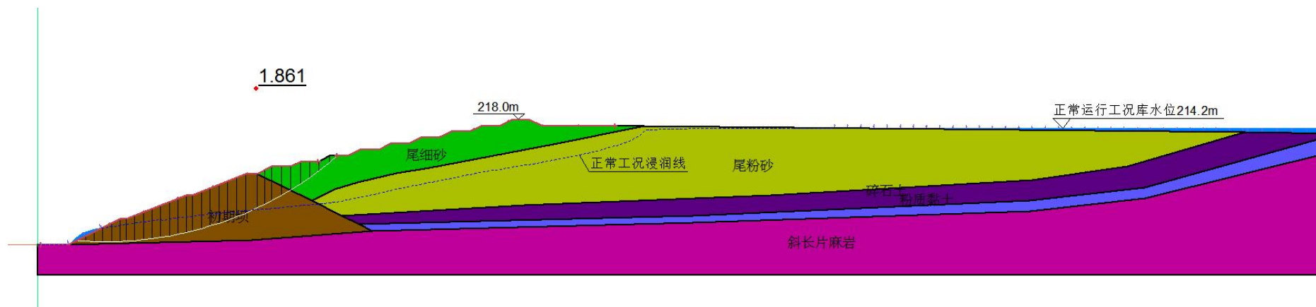
图 3.2-19 尾矿库末期正常运行工况坝体最危险滑动面 ( K_{min}=1.861 )
