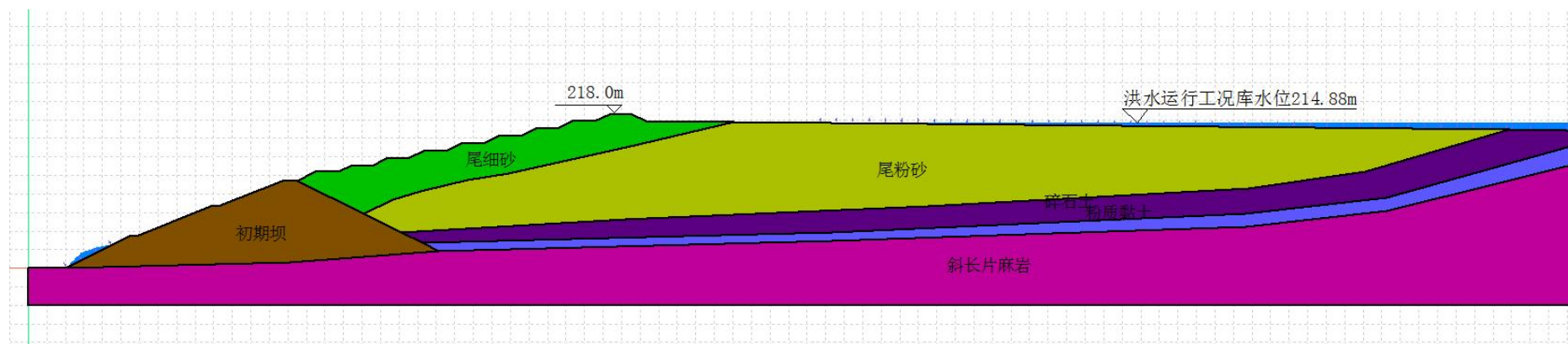
图 3.2-16 尾矿库末期洪水运行工况 214.88m 水位加荷载
