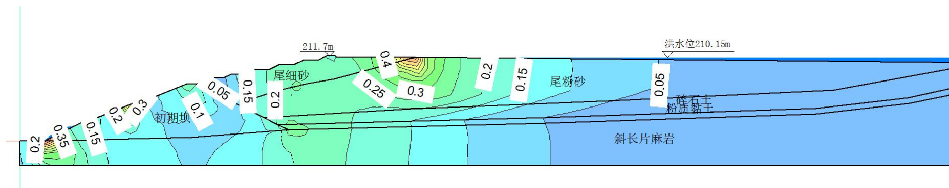
图 3.2-7 尾矿库现状洪水运行工况坝体内部水力梯度计算结果云图
