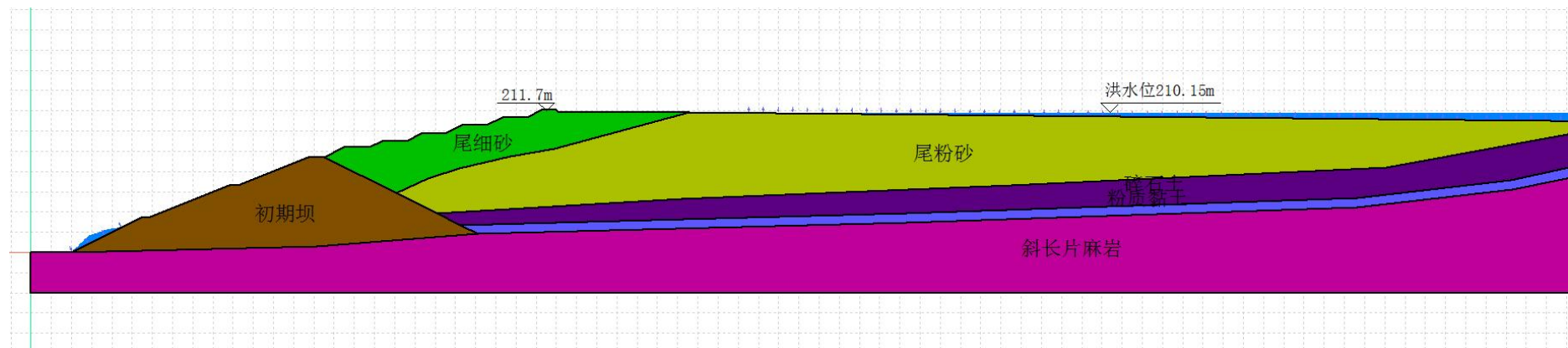
图 3.2-6 尾矿库现状洪水运行工况 210.15m 水位加荷载
