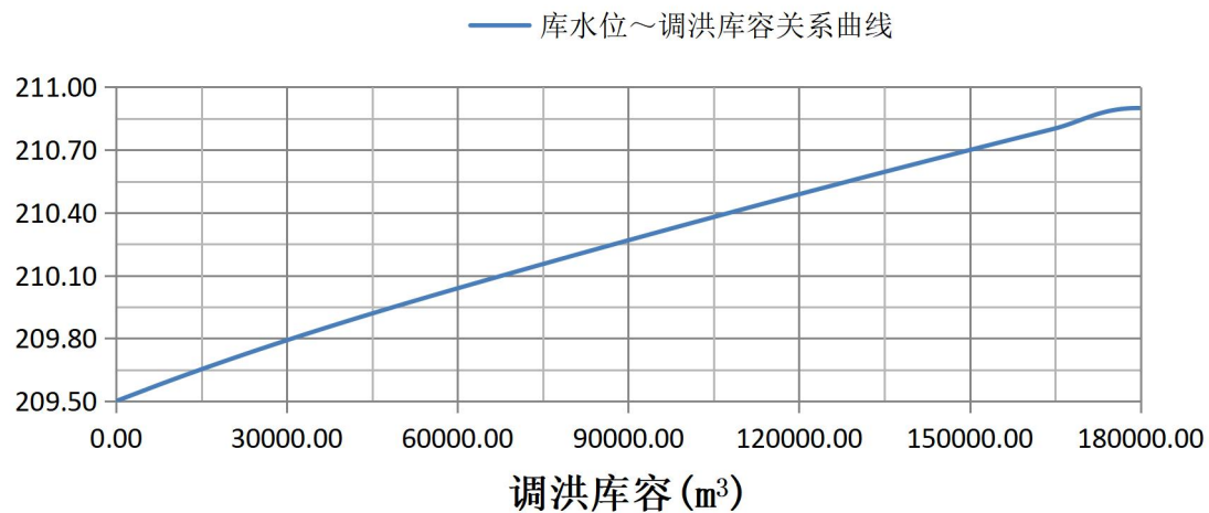
图 3.3-6 库水位~调洪库容关系曲线图
