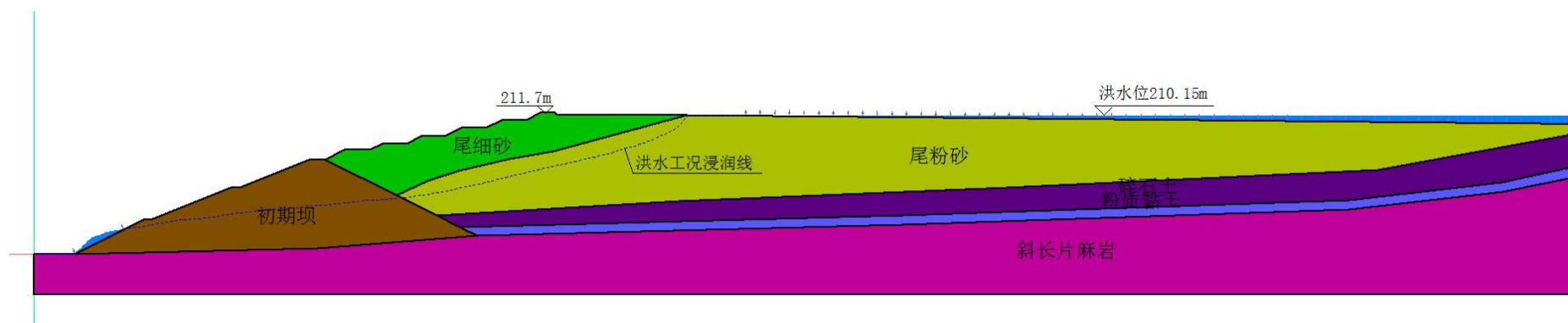
图 3.2-8 尾矿库现状洪水运行工况坝体内部浸润线计算结果云图
