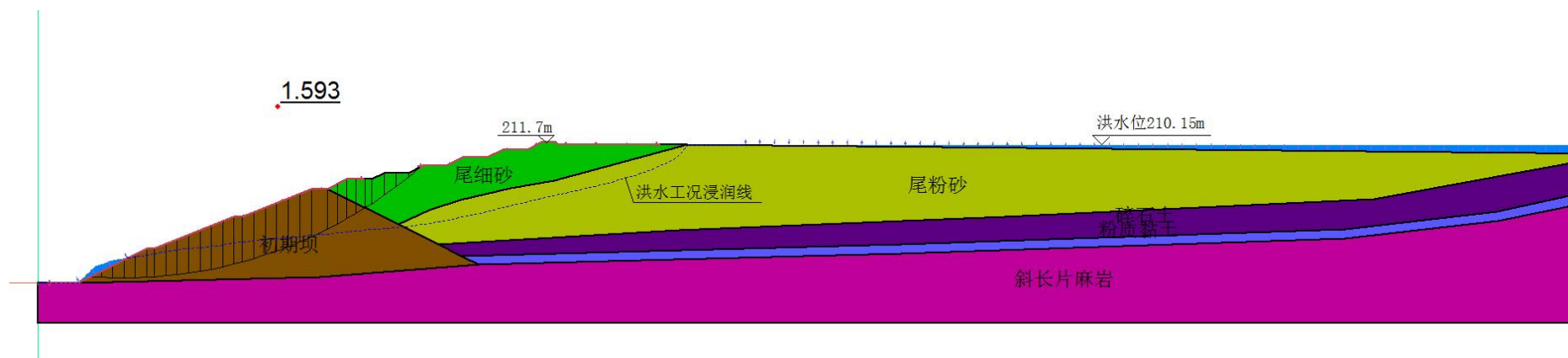
图 3.2-10 尾矿库现状洪水运行工况坝体最危险滑动面 ( K_{min}=1.593 )
