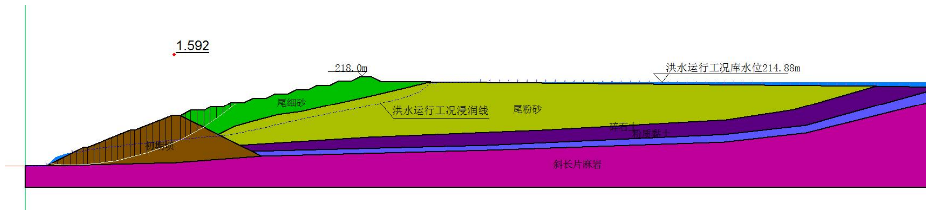
图 3.2-20 尾矿库末期洪水运行工况坝体最危险滑动面 ( K_{min}=1.592 )
