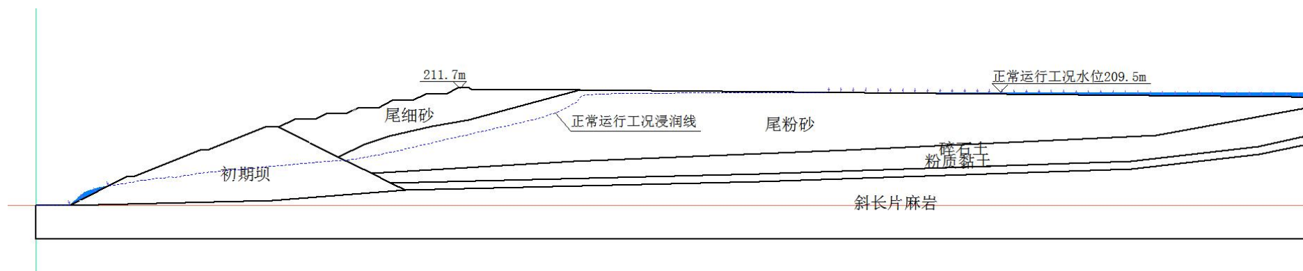
图 3.2-5 尾矿库现状正常运行工况坝体内部浸润线计算结果云图
