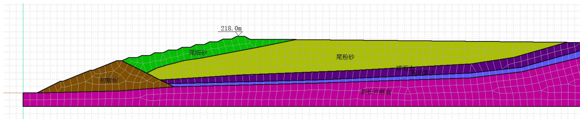
图 3.2-12 尾矿库末期坝体有限元分析网格剖分
