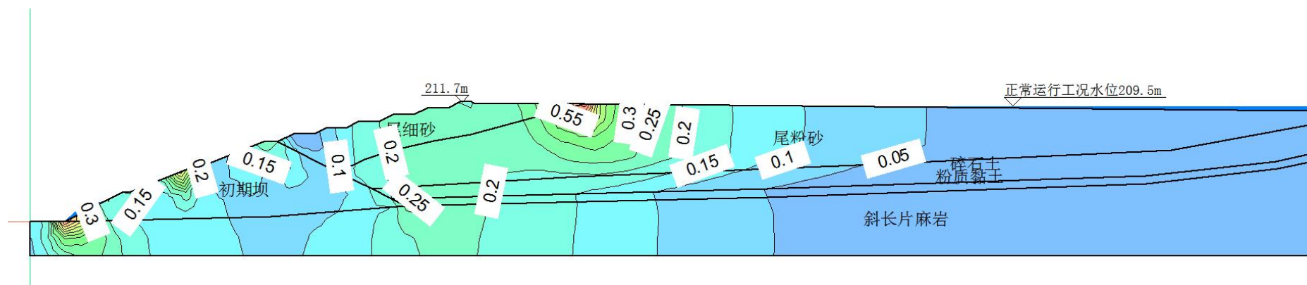
图 3.2-4 尾矿库现状正常运行工况坝体内部水力梯度计算结果云图
