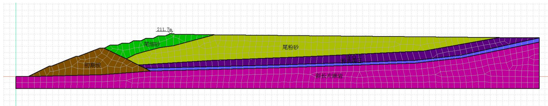
图 3.2-2 尾矿库现状坝体有限元分析网格剖分
