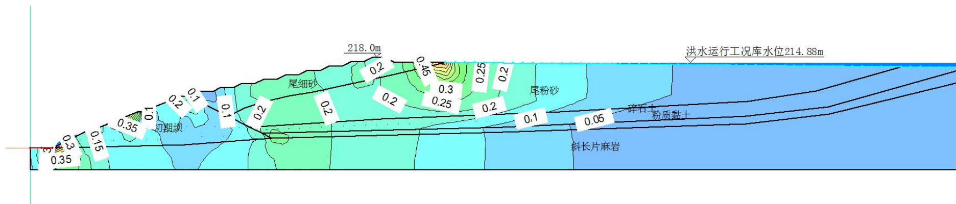
图 3.2-17 尾矿库末期洪水运行工况坝体内部水力梯度计算结果云图
