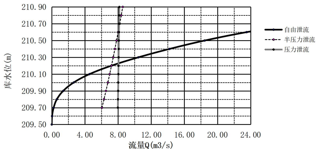
图 3.3-5 排水斜槽排水系统库水位与泄流量关系曲线图
