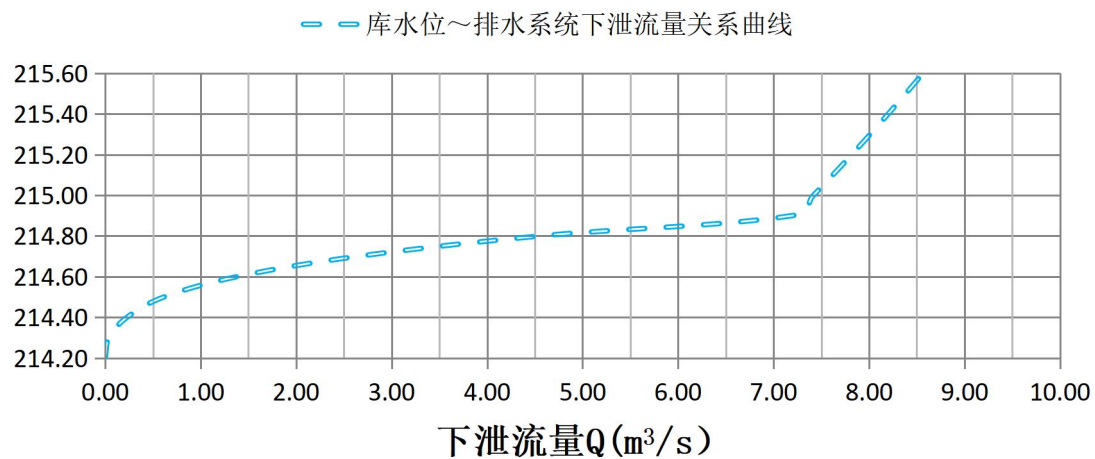
图 3.3-12 库水位与下泄流量关系曲线图
