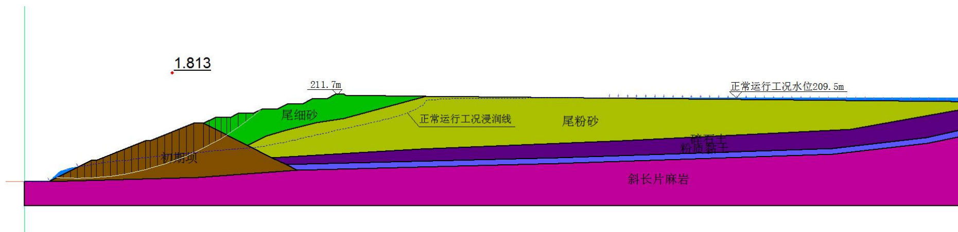
图 3.2-9 尾矿库现状正常运行工况坝体最危险滑动面 ( K_{min}=1.813 )
