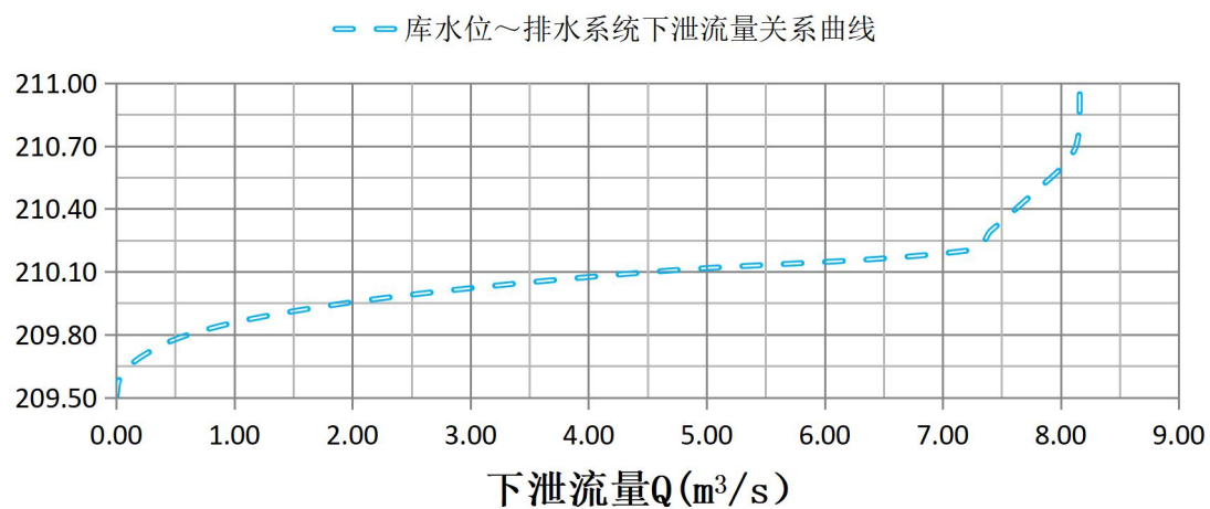
图 3.3-7 库水位~下泄流量关系曲线图
