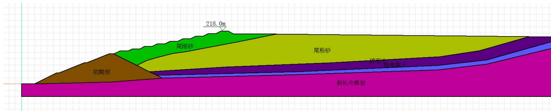
图 3.2-11 尾矿库末期坝体渗流分析计算模型
